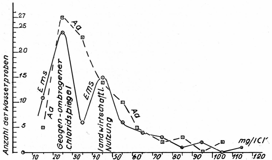
Abb. 3 Häufigkeitskurven des Chlorid-Gehaltes in Gewässern
