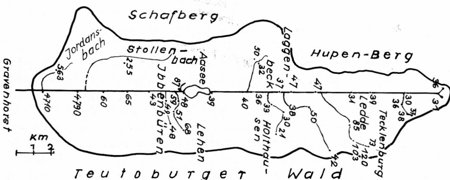
Abb. 5 Der Chlorid-Stammbaum der Ibbenbürener Aa bezogen auf die ehemalige Klosterkirche in Gravenhorst
