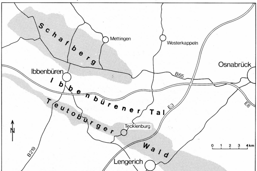
Abb. 1 Das Ibbenbürener Tal zwischen Schafberg im N und Teutoburger Wald im S
