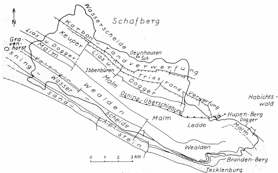
Abb. 2 Das Einzugsgebiet des Ibbenbürener Tales bezogen auf Gravenhorst (Klosterkirche) mit Darstellung des mesozoischen Sockels unter Eintragung der Wasserscheiden (Unterlagen: Geol. Karten 1:25 000 Bl. 3911 Hopsten, 3711 Bevergern, 3712 Tecklenburg, 3713 Hasbergen, Preußag Kohle AG Steinkohlenbergwerke Ibbenbüren nebst eigenen Aufnahmen)
